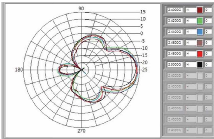
Horizontal Pattern H-plane
